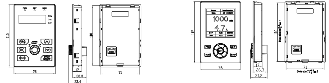
GT35-LKD键盘尺寸 (单位: mm)
