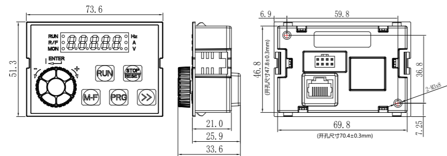
GT35LKD-A键盘尺寸(GT35-4T0007P~GT35-4T0022P) (单位: mm)
