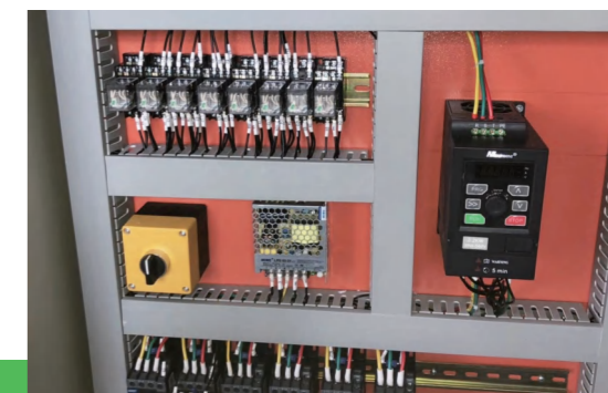
变频器在新风系统上的应用
