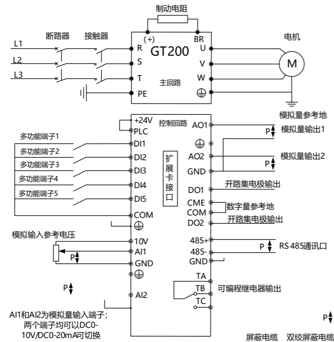
适用机型: GT200-4T0300G/4T0370P-B及以下
