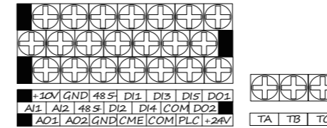
GT200-4T0055G/4T0075P-B及以下控制板端子排列顺序图
