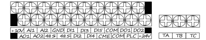
GT200-4T0055G/4T0075P及以上控制板端子排列顺序图
