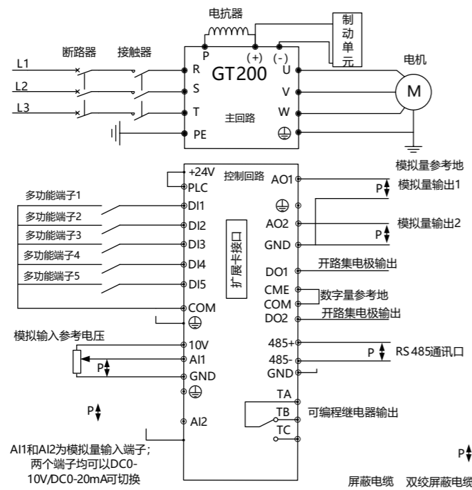
适用机型: GT200-4T0300G/4T0370P及以上
