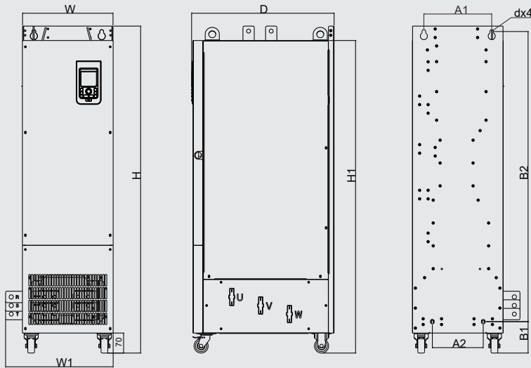
SIZE J 外形尺寸及安装尺寸样式示意图
