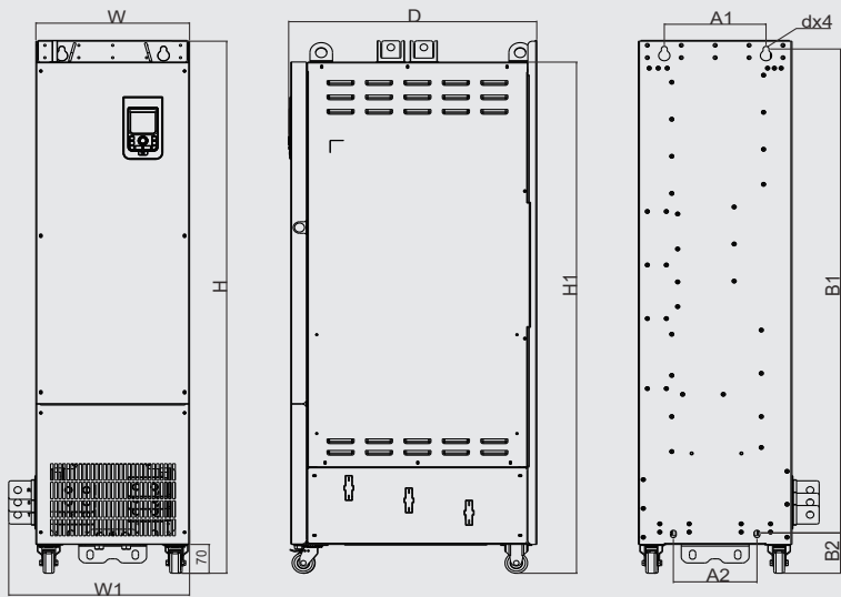
SIZE K 外形尺寸及安装尺寸样式示意图
