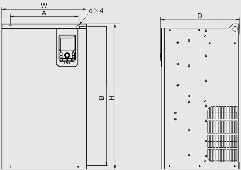
SIZE G~SIZE I 外形尺寸及安装尺寸样式示意图
