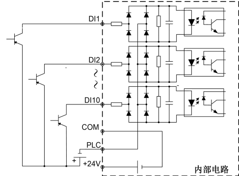
图 2-29 外部电源供电 PNP 图（OE）
