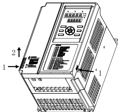
图 2-10 盖板的拆卸
