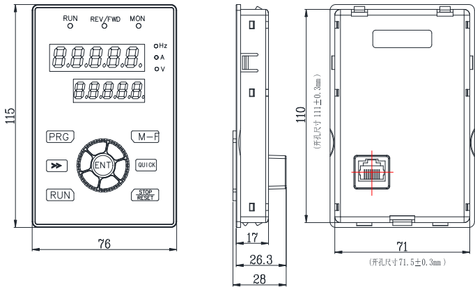
图 1-1 GT200-LKD 键盘尺寸（GT200-2S0007G~GT200-4T8500G）
