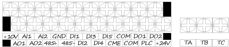
图 2-20 GT200-4T0055G/4T0075P 及以上控制板端子排列顺序图
