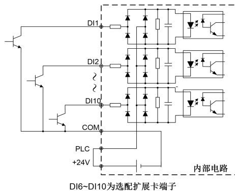
图 2-26 内部电源供电 NPN 图 (OC)
