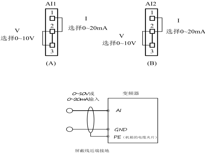
图2-21 模拟输入端子配线
