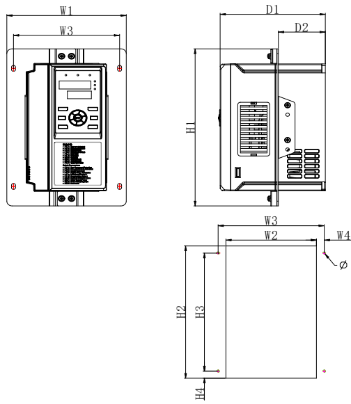
(1) 塑胶结构嵌入式安装支架规格尺寸
