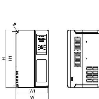
(a1) A1 规格尺寸
