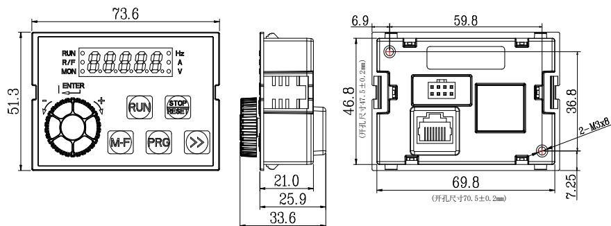
图 1-2 GT200-LKD-A 键盘尺寸 (GT200-4T0007G-B~GT200-4T0040G-B)
